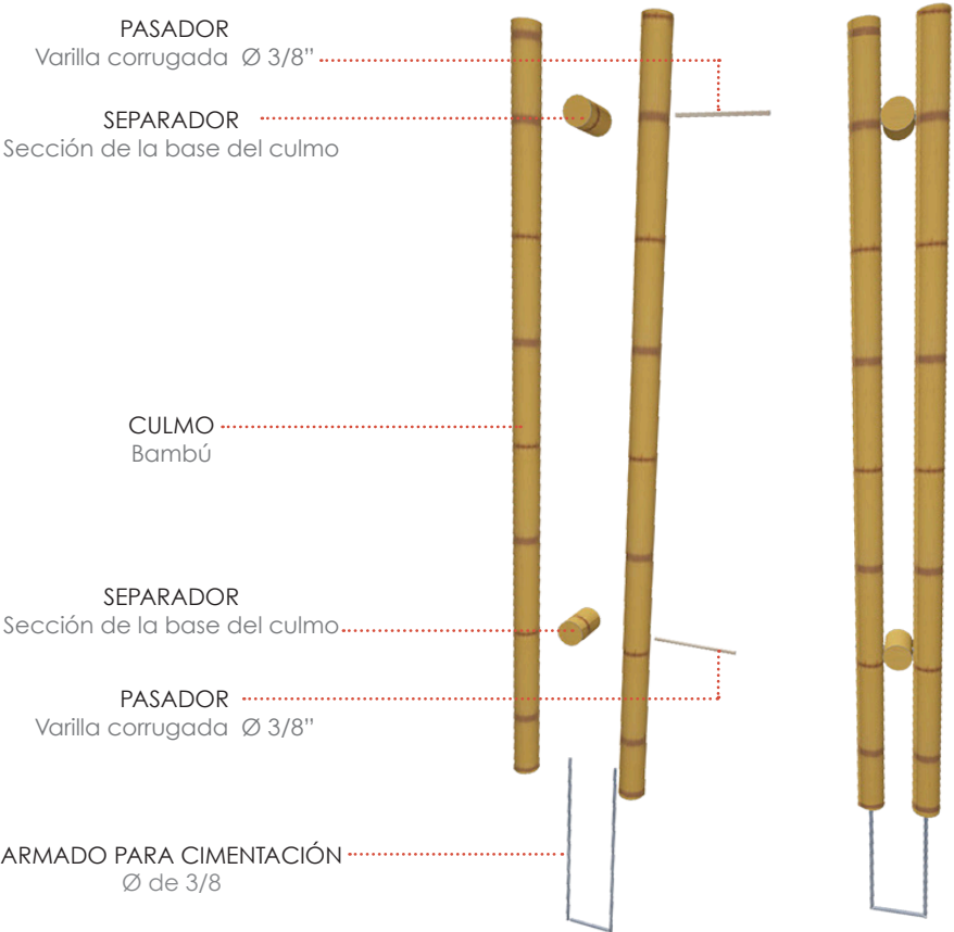
Isométrico
