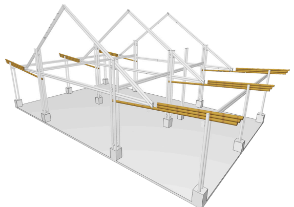
V-4 Vigas de Pórtico 6 vigas
