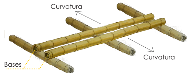
Fig. 3.6. Orientación de las curvas.
